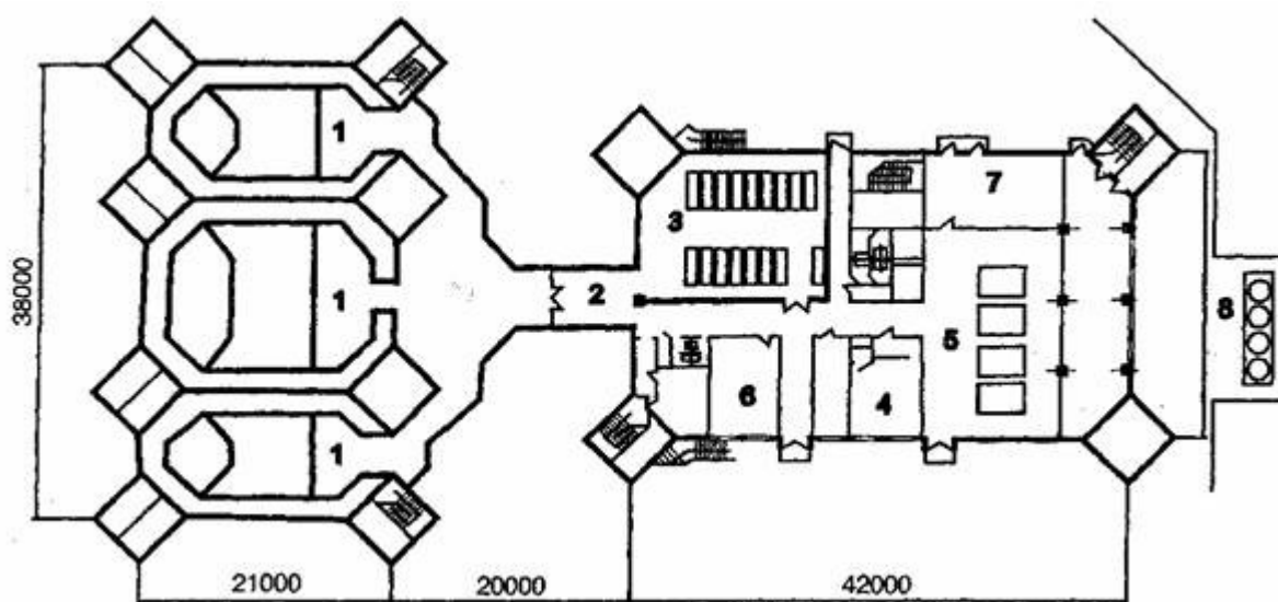
Рисунок 7 — Проект крематория в Ростове-на-Дону
